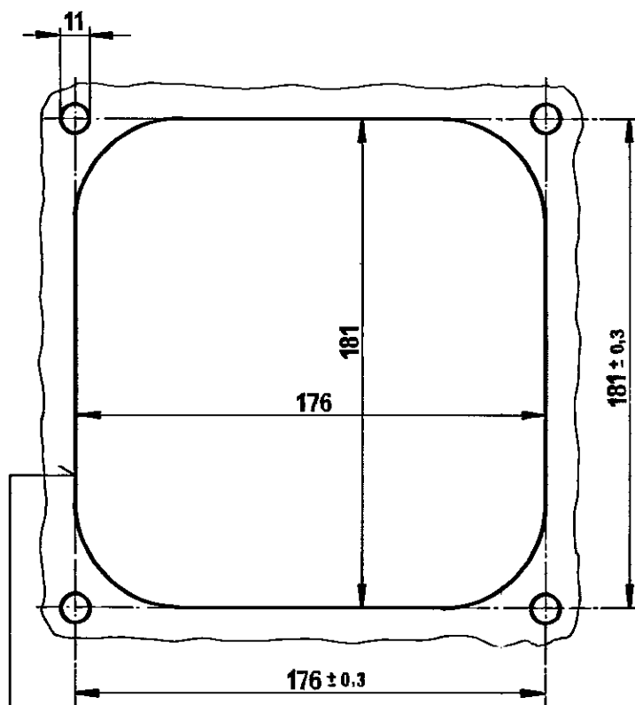
Erforderlicher Ausschnitt zum Einbau der Anzeigevorrichtung
