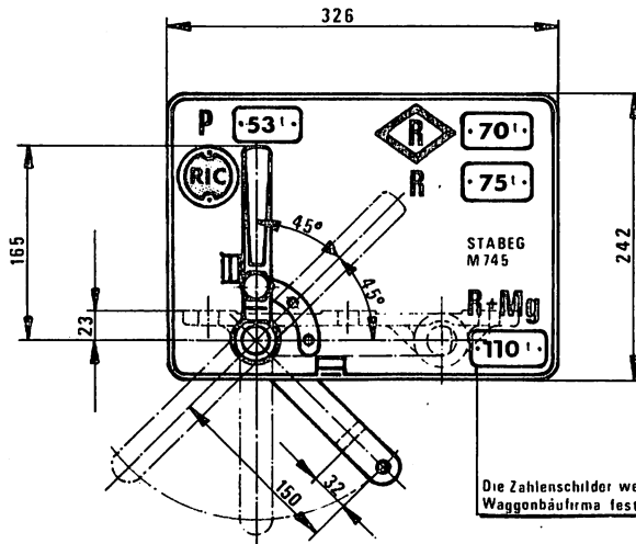
Ansicht A
