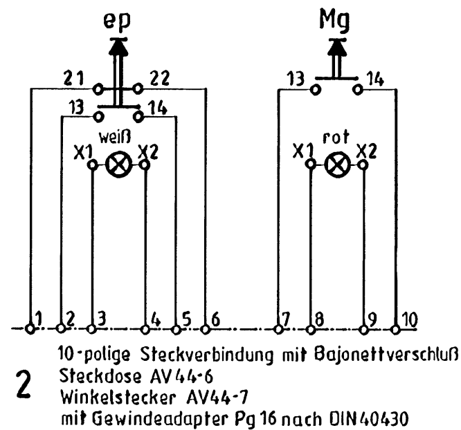
Elektr. Schema für Anzeigevorrichtung AV 440
